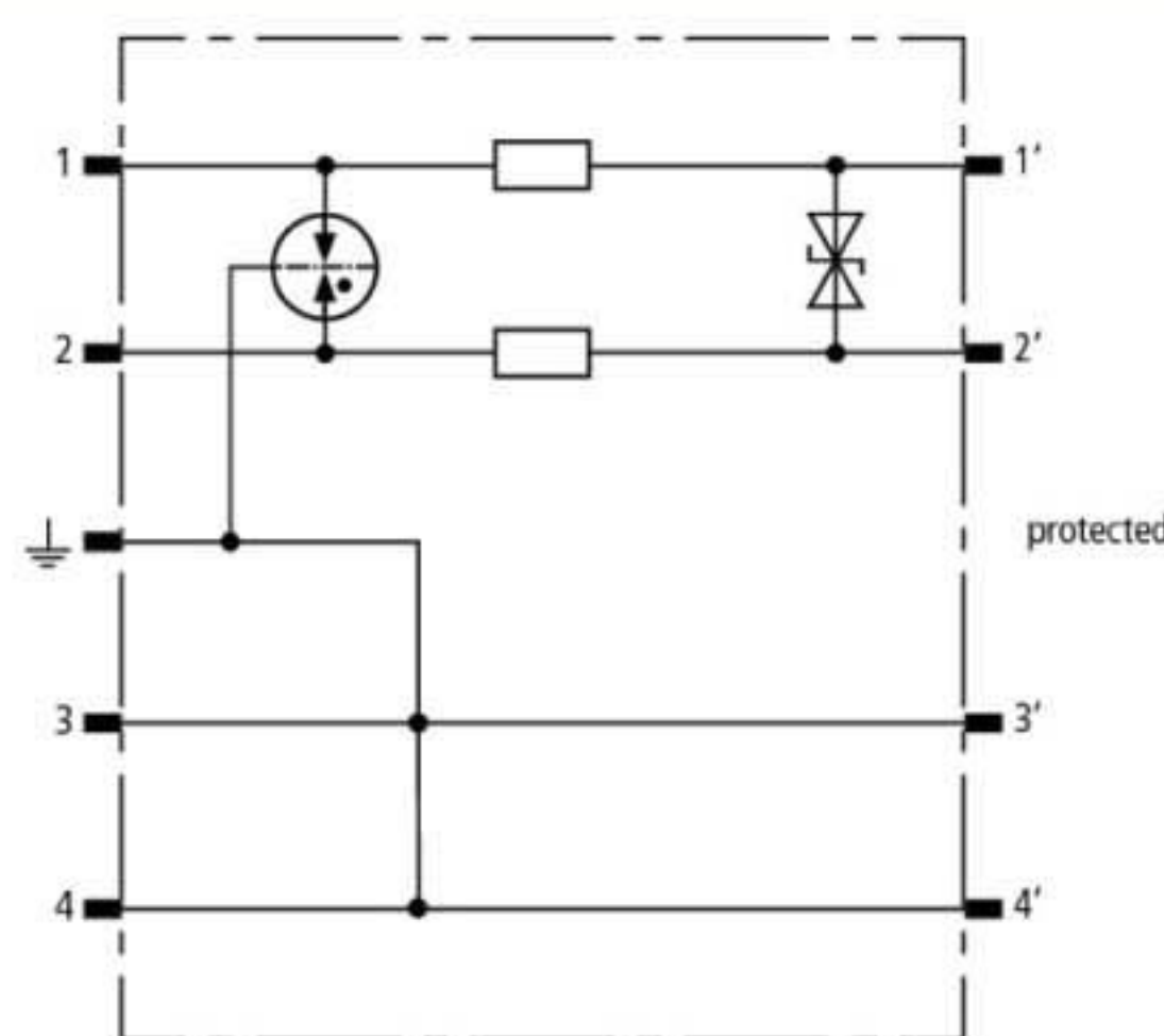
Принципиальная схема BSP M2 BD 180
