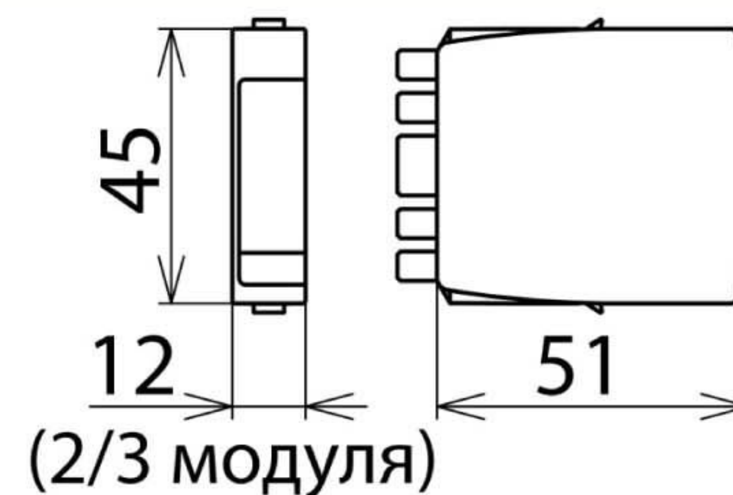
Размерный эскиз BSP M2 BD 180
