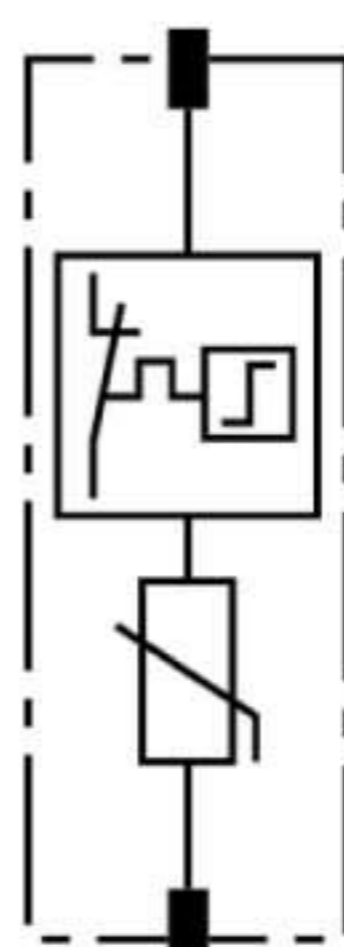
Принципиальная схема DG MOD 440
