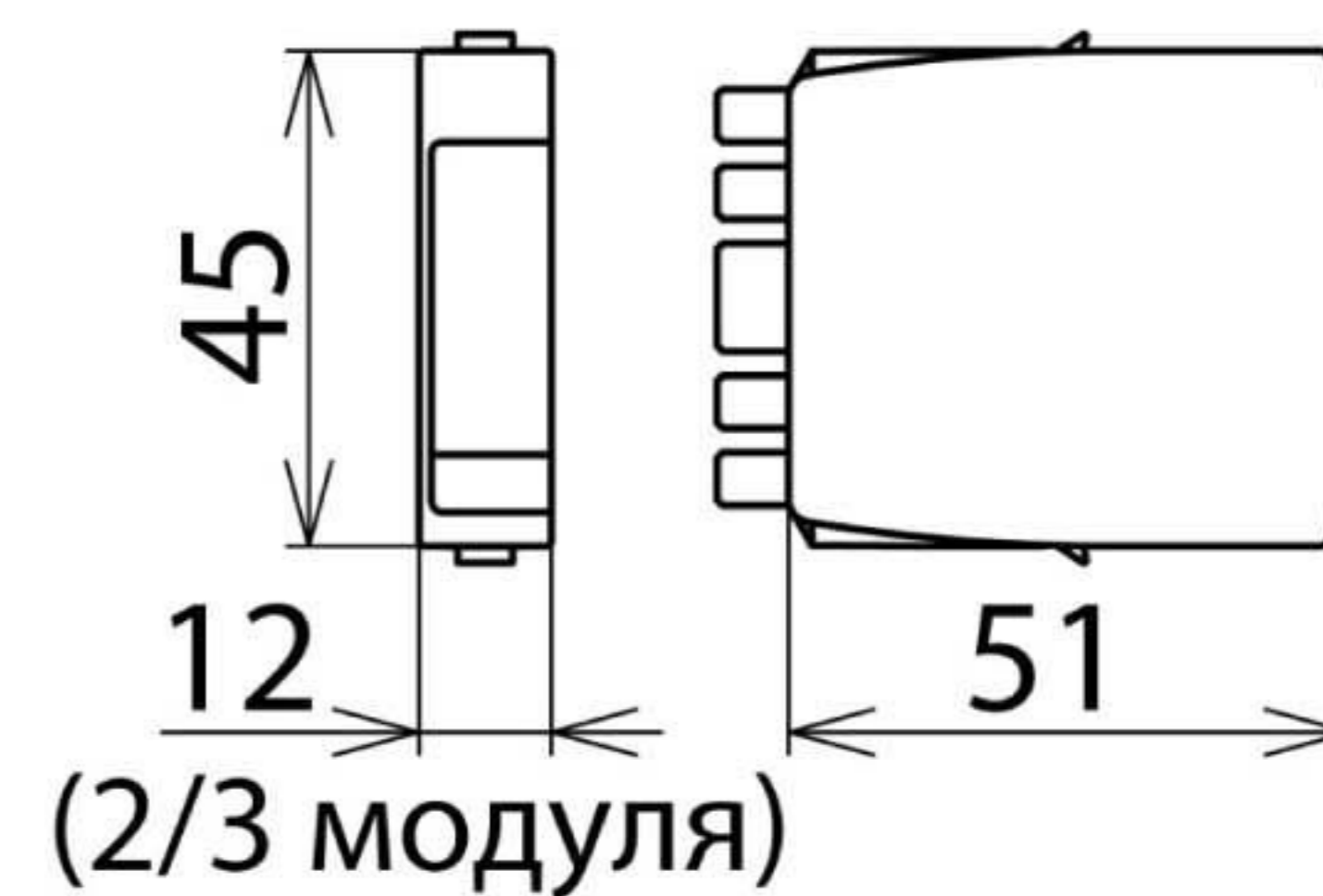
Размерный эскиз ВХТ М4 Е
