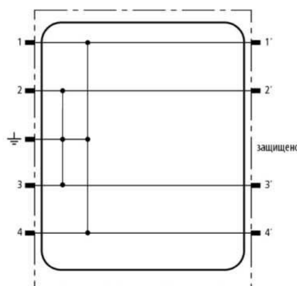
Принципиальная схема ВХТ М4 Е
