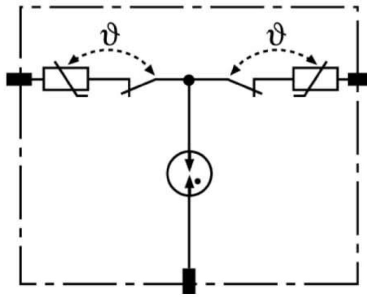
Принципиальная схема DR MOD 30
