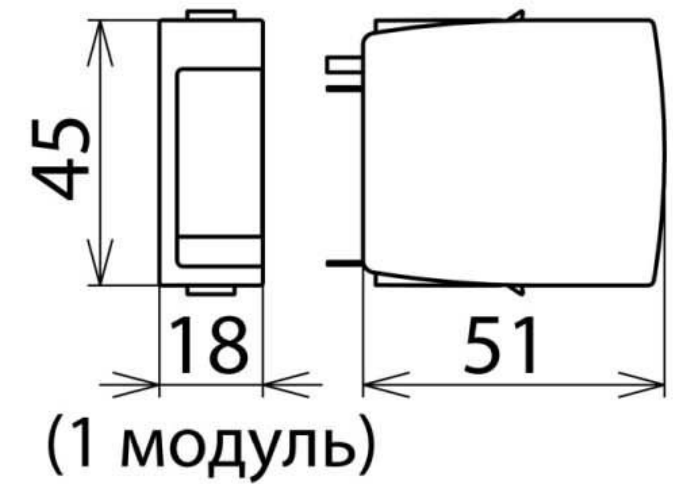
Размерный эскиз DR MOD 30
