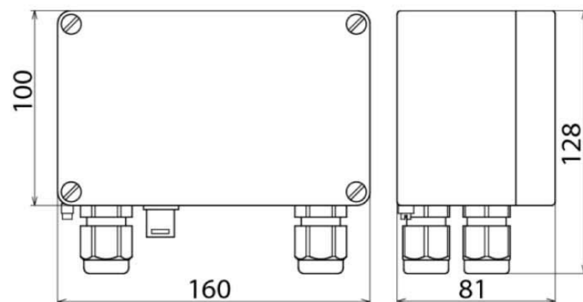
Размерный эскиз ALGA 5 X
