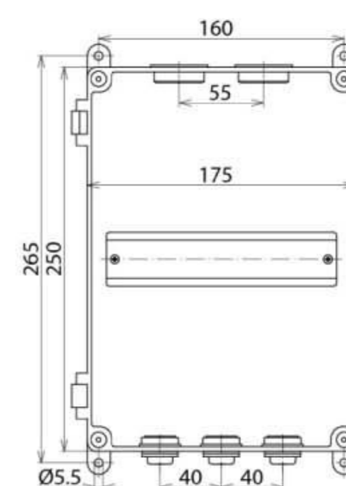
Размерный эскиз IGA 7 IP54
