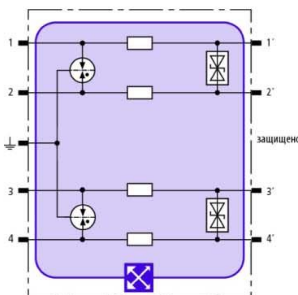
Принципиальная схема BXT ML4 BD HF 5
