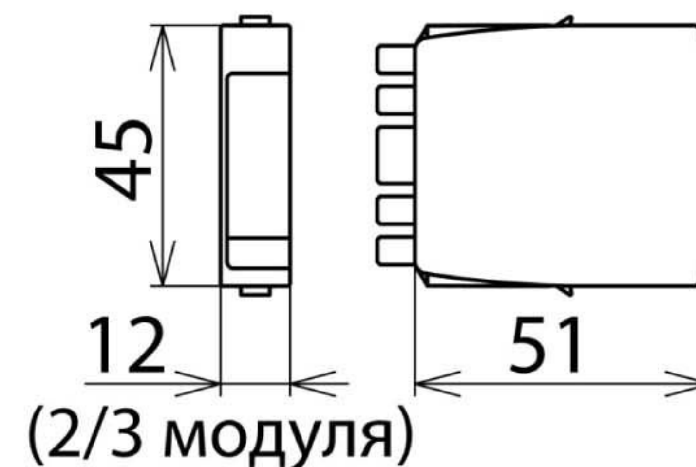
Размерный эскиз BXT ML4 BD HF 5
