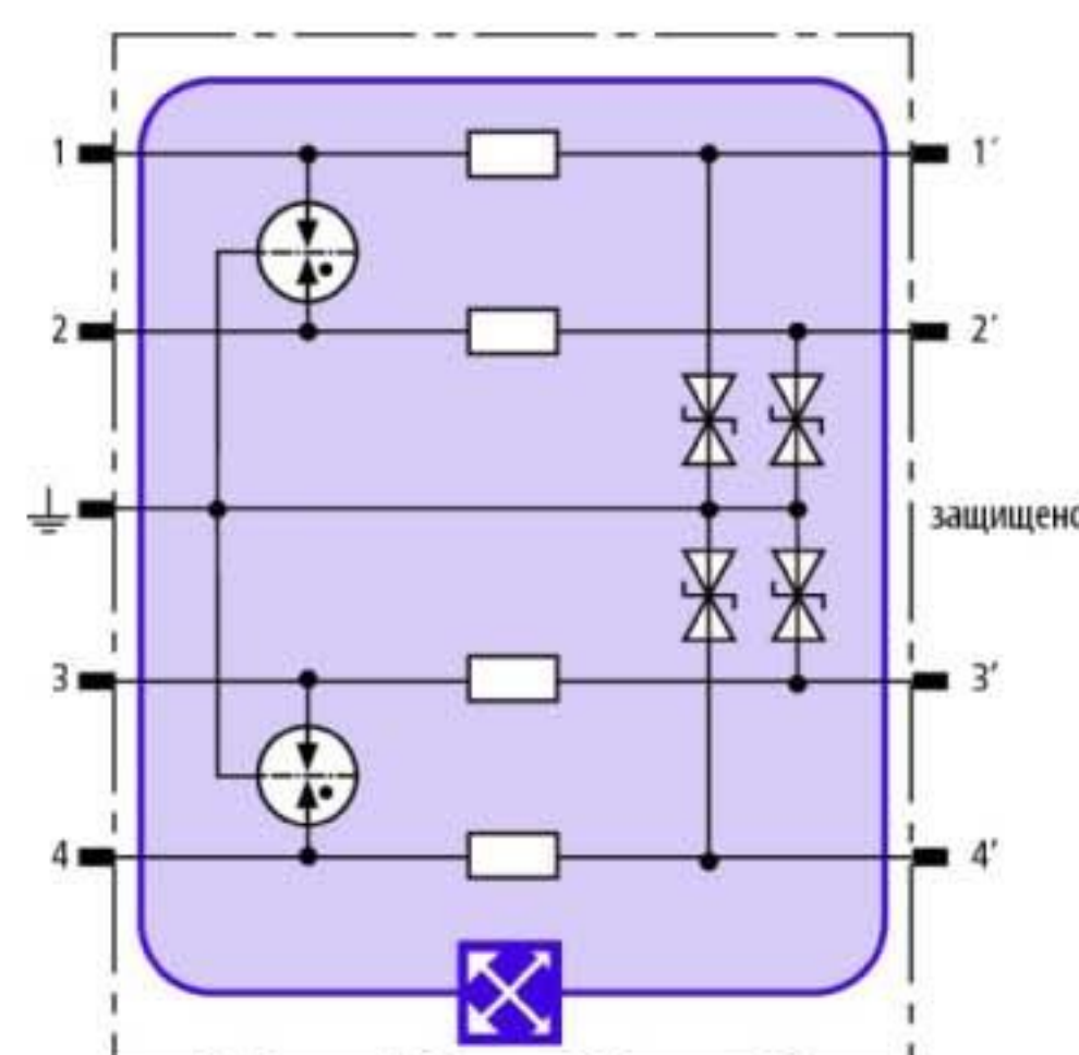
Принципиальная схема BXT ML4 BE 24
