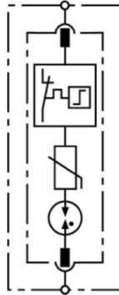
Принципиальная схема DG S 75 VA
