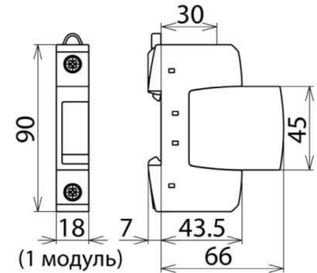
Размерный эскиз DG S 75 VA
