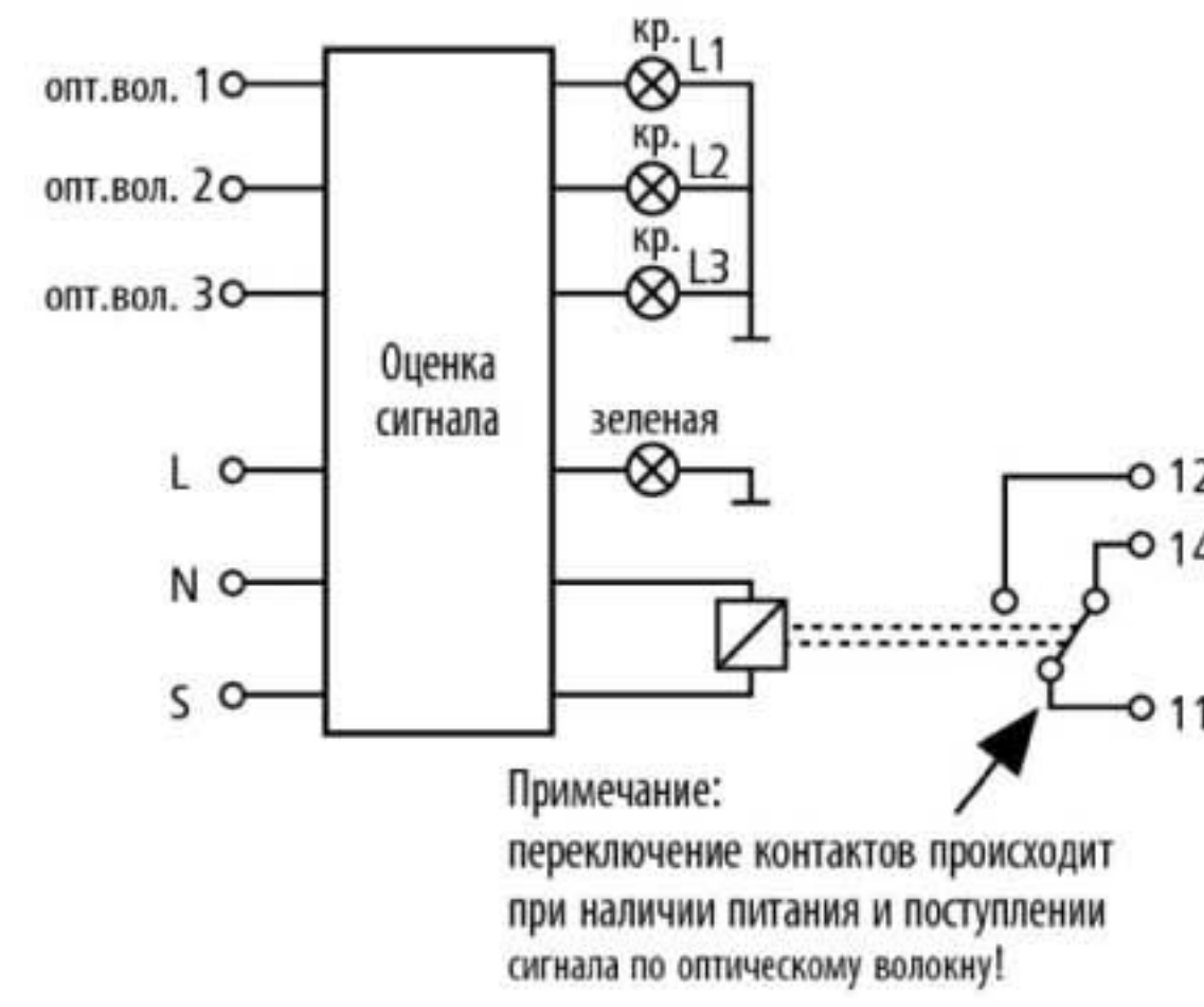
Принципиальная схема DSI E 3
