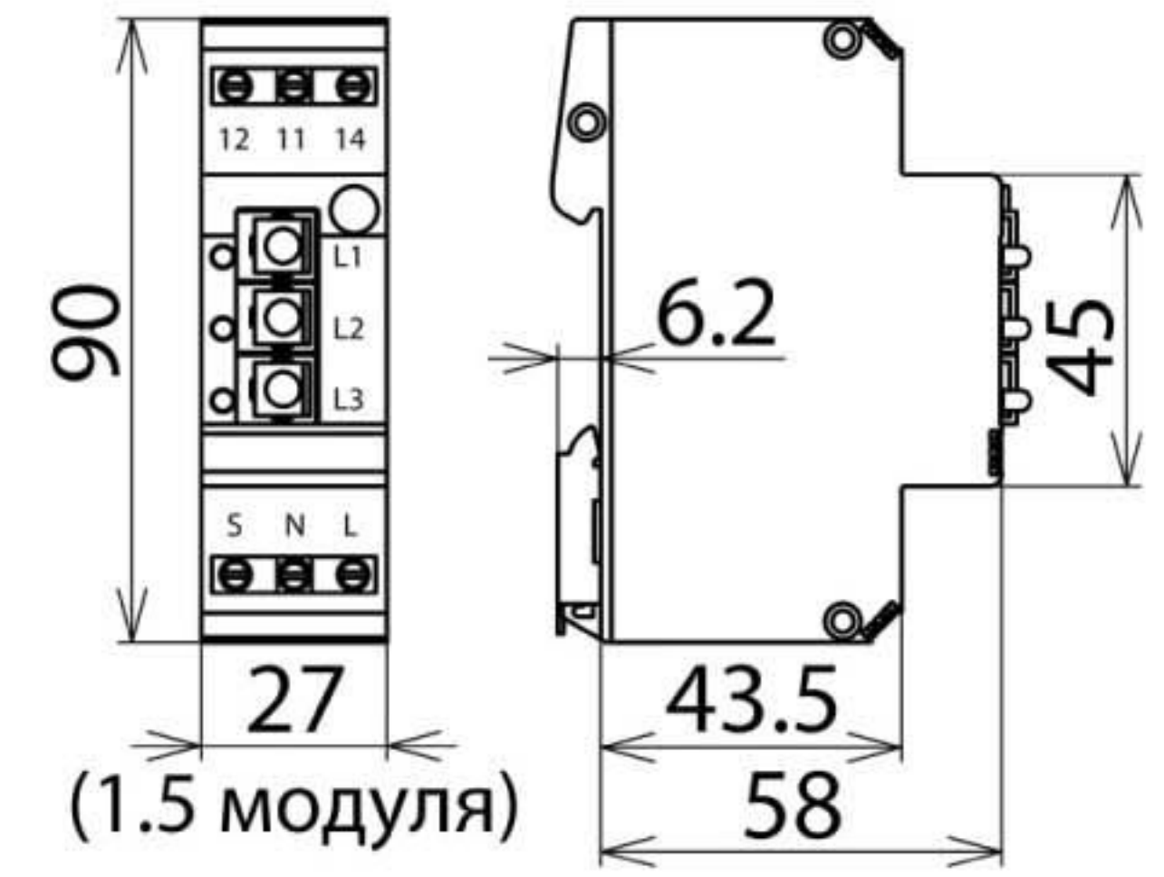
Размерный эскиз DSI E 3
