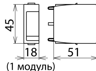
Размерный эскиз DG MOD PV SCI 500
