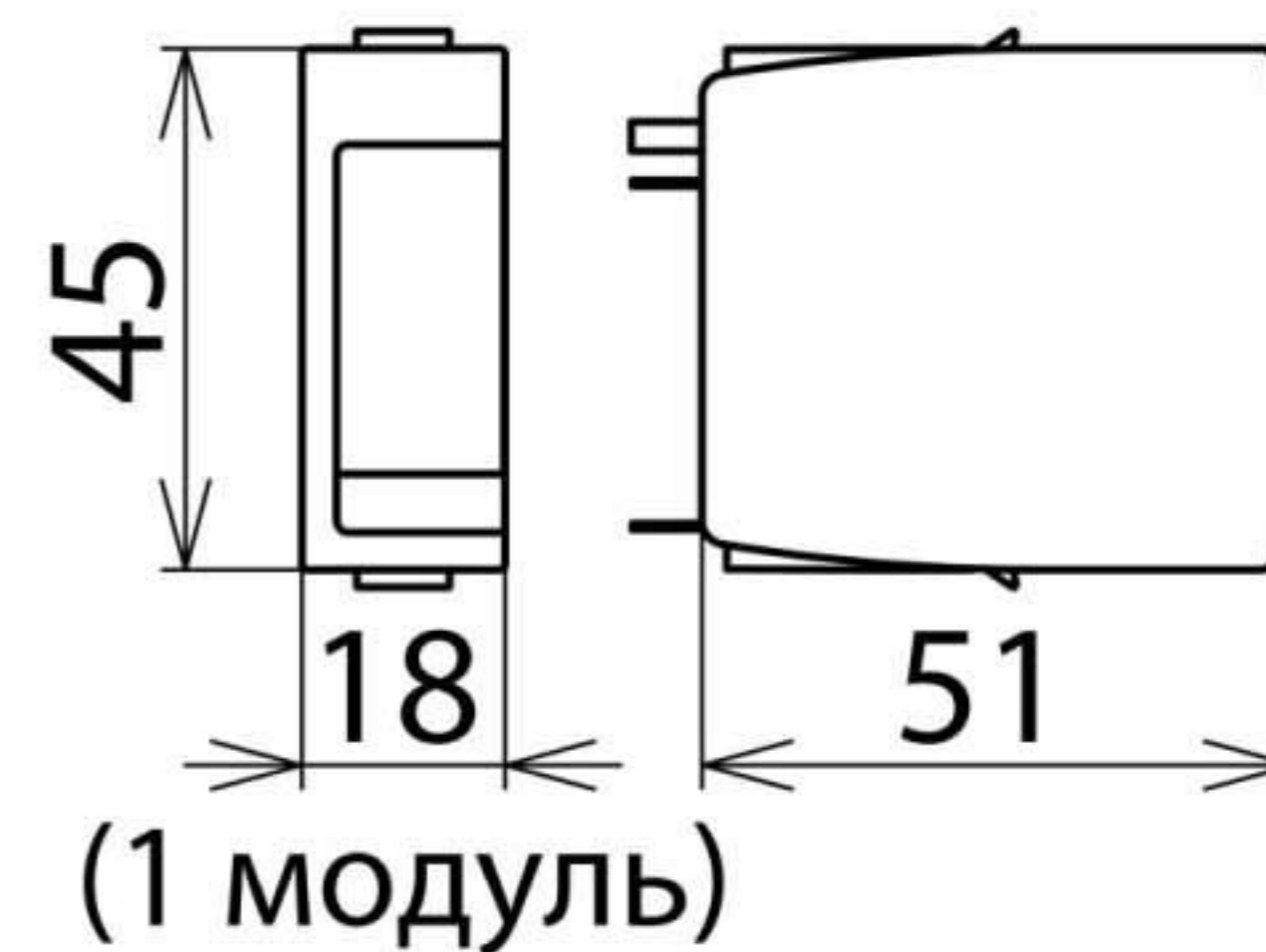
Размерный эскиз DR MOD 60
