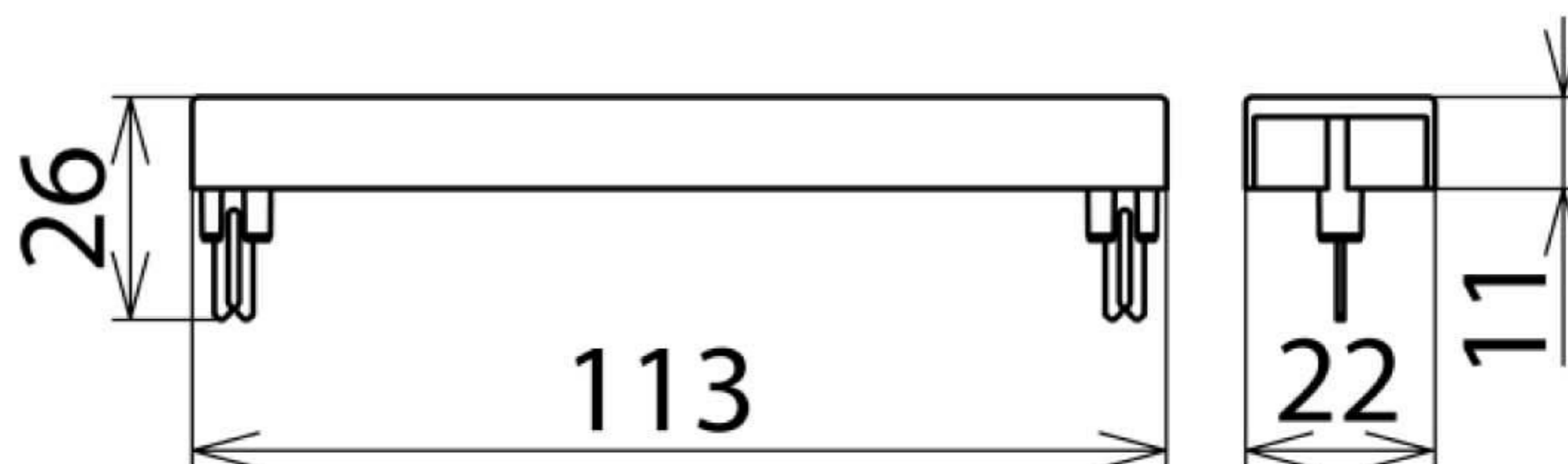
Размерный эскиз EF 10 DRL
