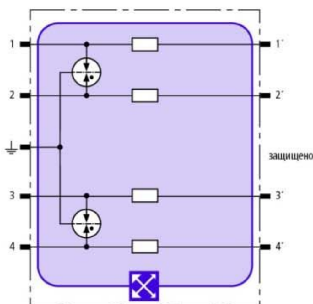
Принципальная схема BXT ML4 B 180
