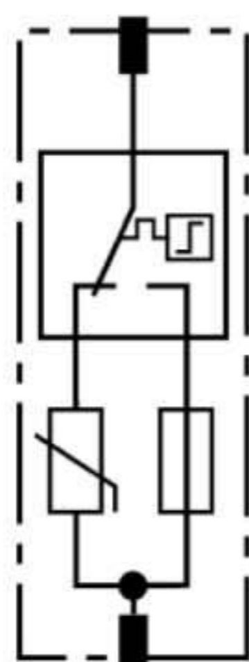
Принципиальная схема DG MOD E PV SCI 750
