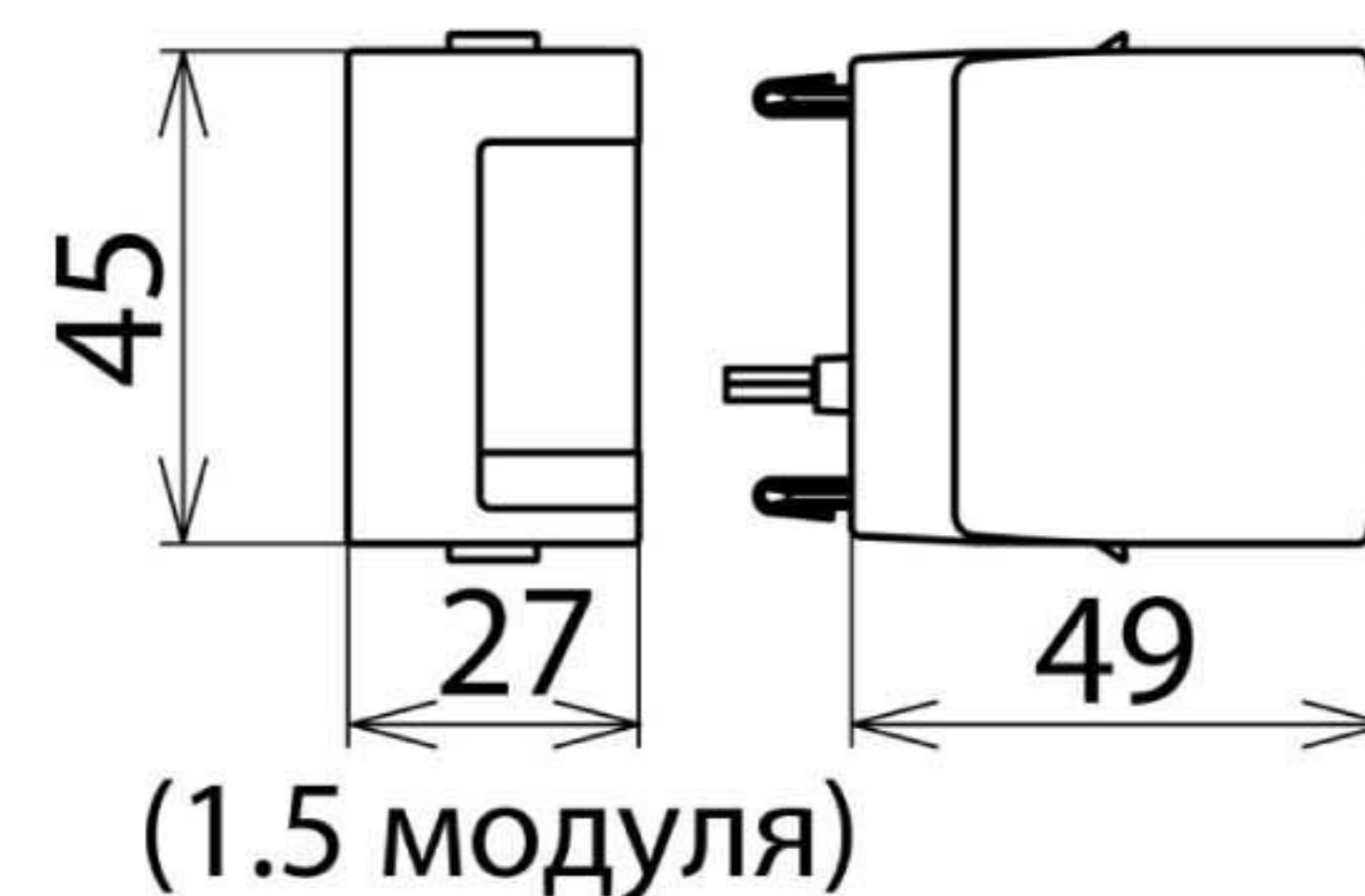
Размерный эскиз DG MOD E PV SCI 750
