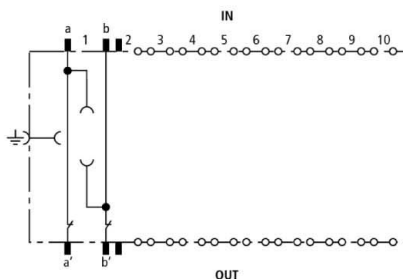
Принципиальная схема BM 10 DR
