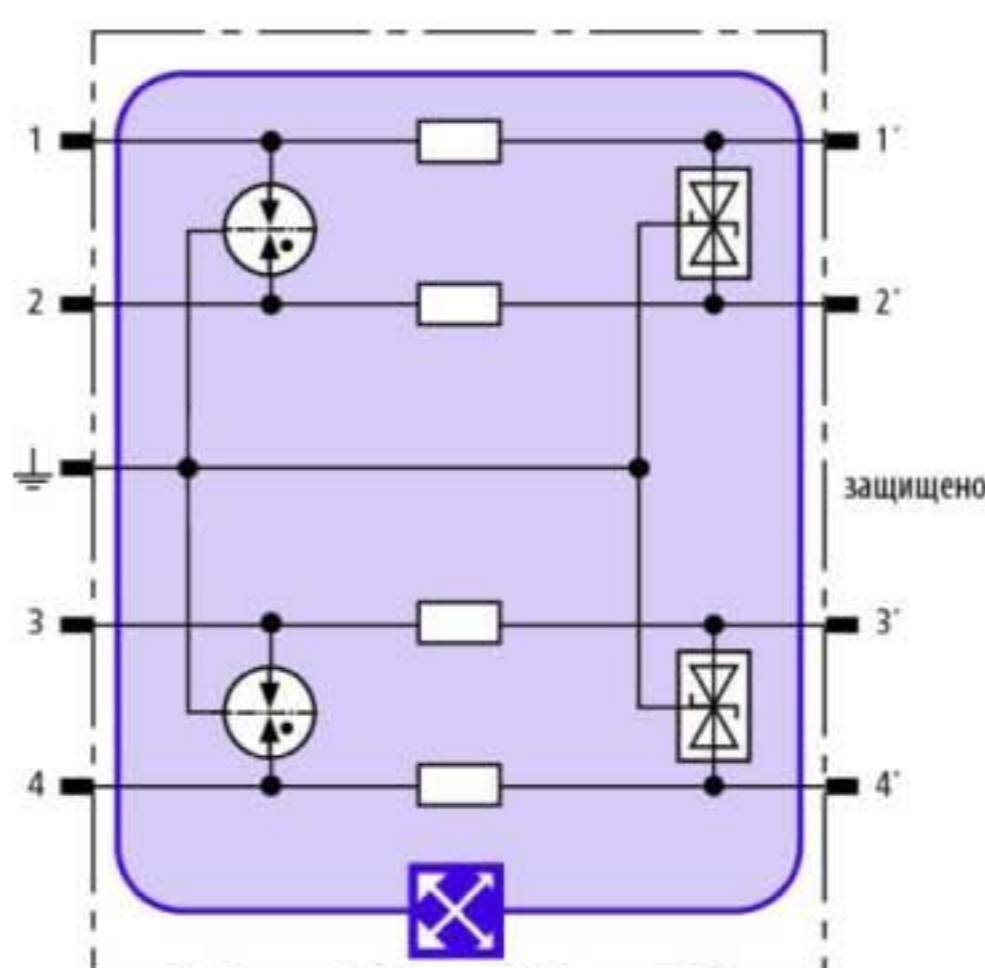
Принципиальная схема BXT ML4 BE HF 5
