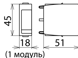
Размерный эскиз DG MOD PV SCI 600
