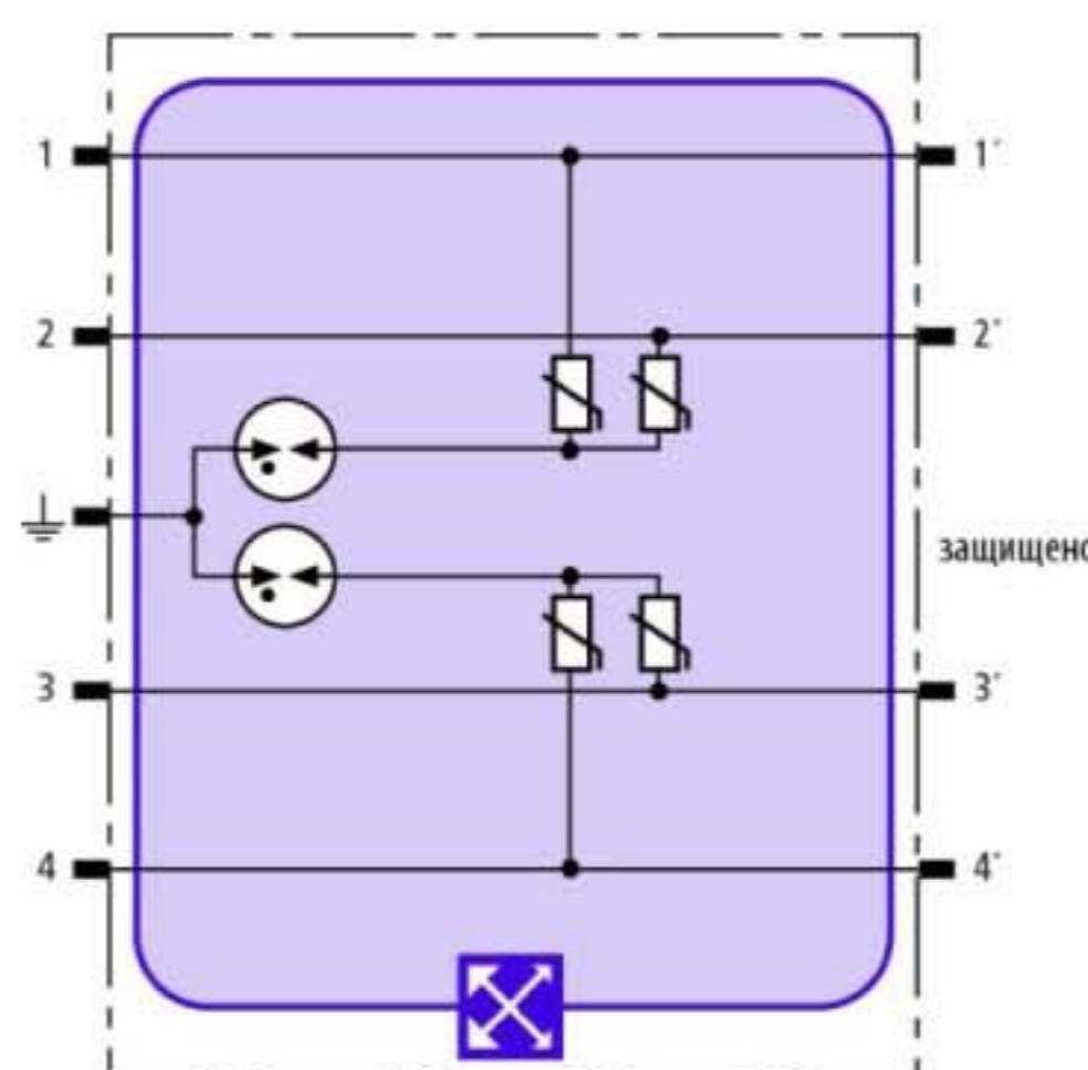
Принципиальная схема VXT ML4 MY 250
