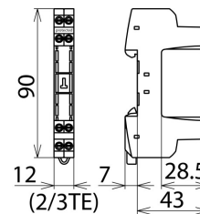
Размерный эскиз BSP BAS 4
