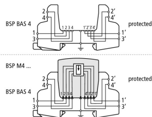
Принципиальная схема соединений с установленным защитным модулем и без него
