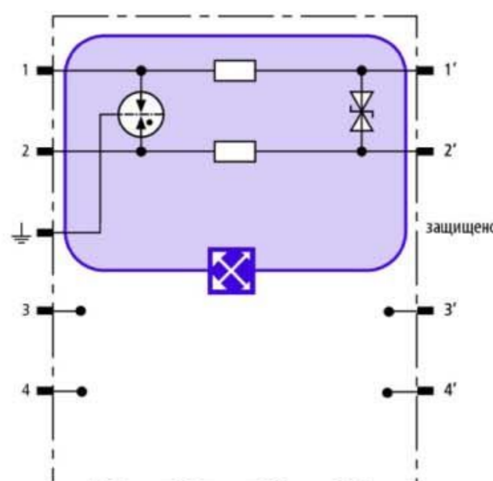
Принципиальная схема BXT ML2 BD 180
