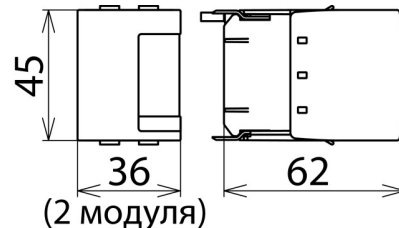
Размерный эскиз DSE MOD 220
