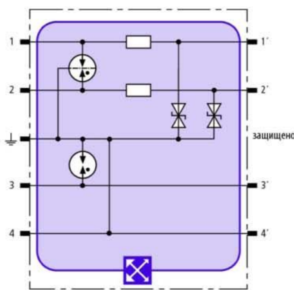
Принципиальная схема BXT ML2 BE S 24
