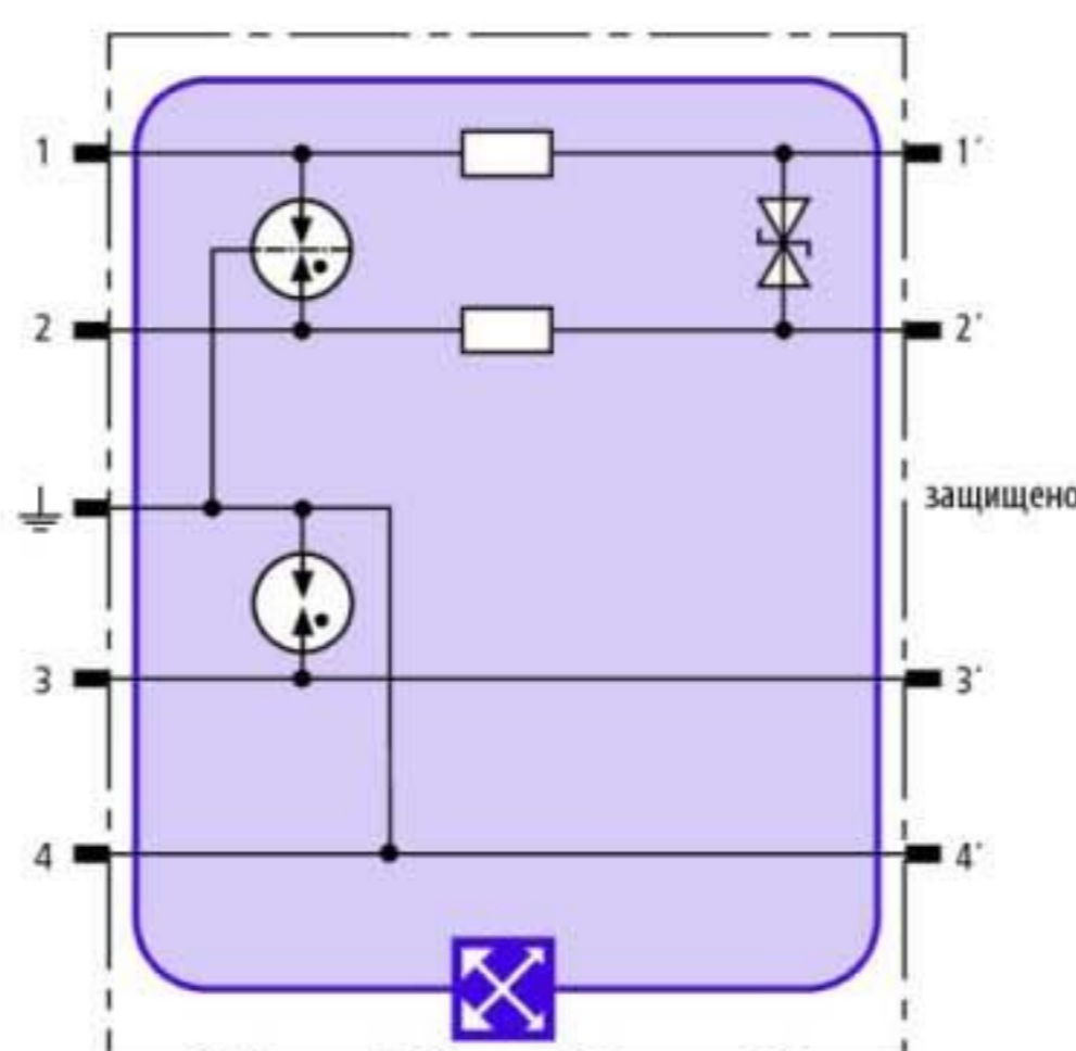
Принципиальная схема BXT ML2 BD S 48
