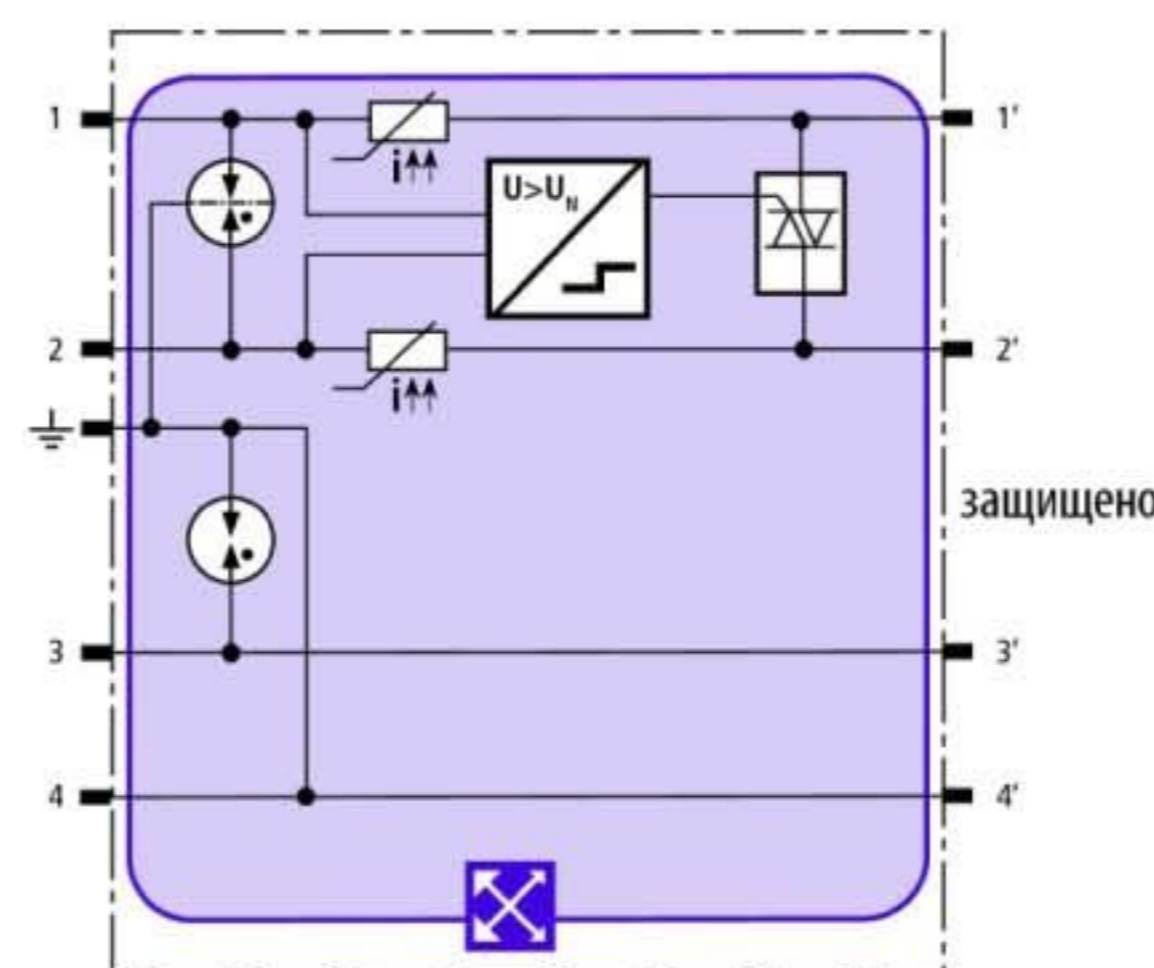
Принципиальная схема BXTU ML2 BD S 0-180
