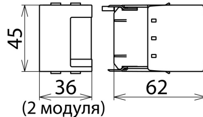
Размерный эскиз DSE MOD 60
