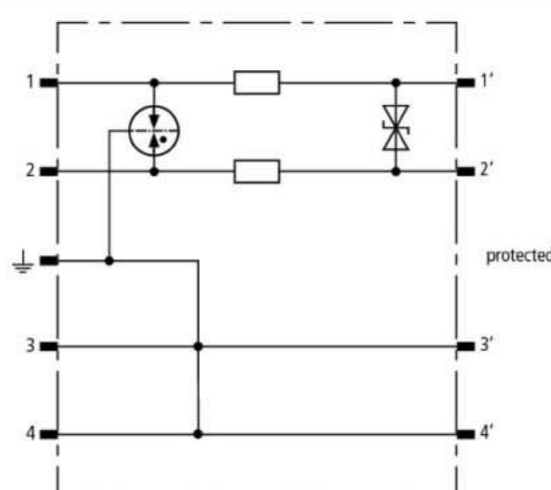
Принципиальная схема BSP M2 BD 60
