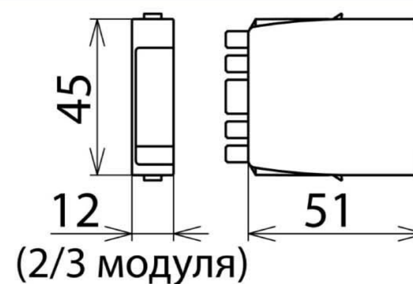
Размерный эскиз BSP M2 BD 60
