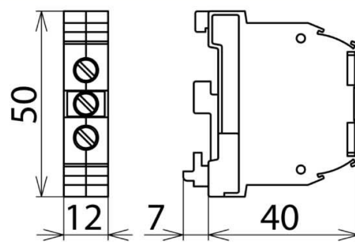
Размерный эскиз SLK 16
