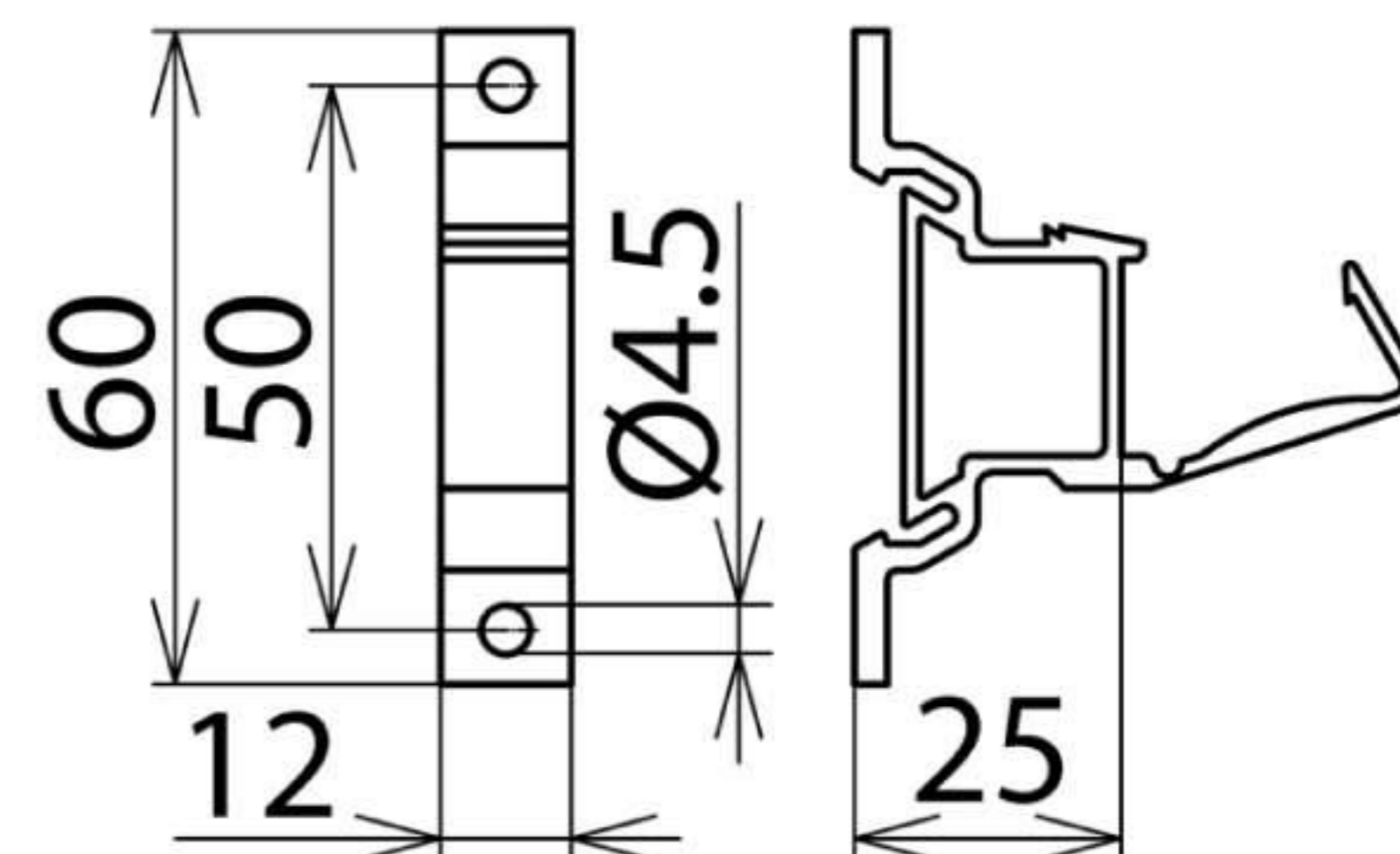
Размерный эскиз SH 18X3 K
