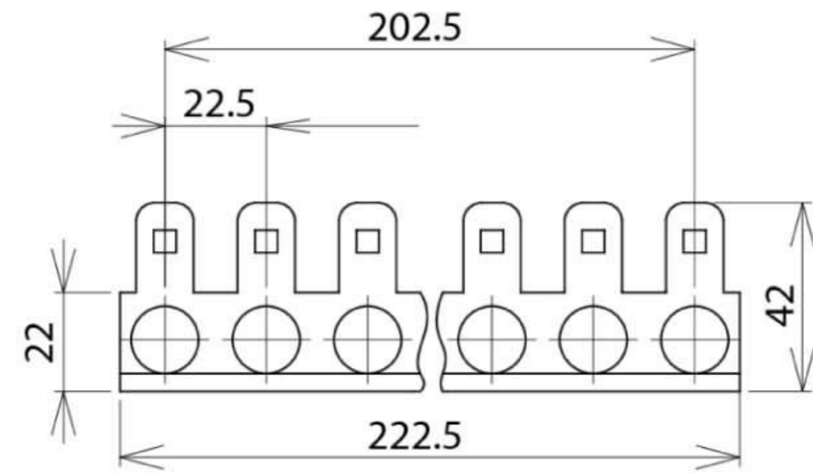
Размерный эскиз MB2 10 LSA
