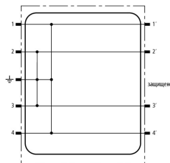
Принципиальная схема ВХТ М4 Е
