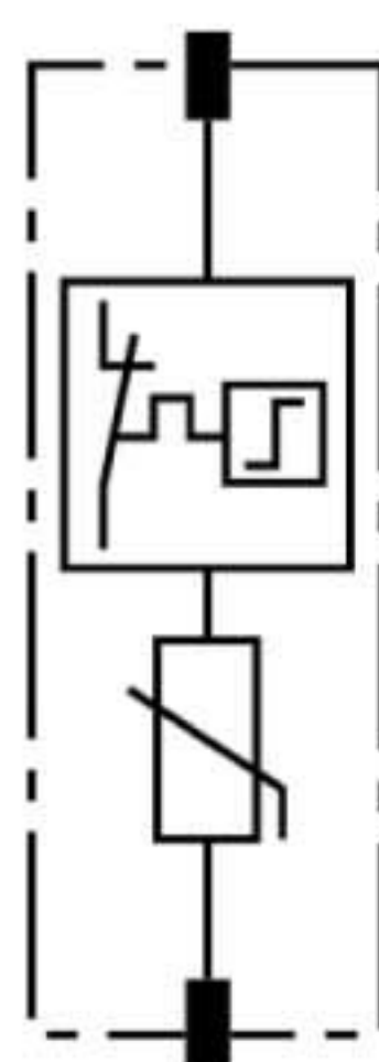
Принципиальная схема DG MOD 150
