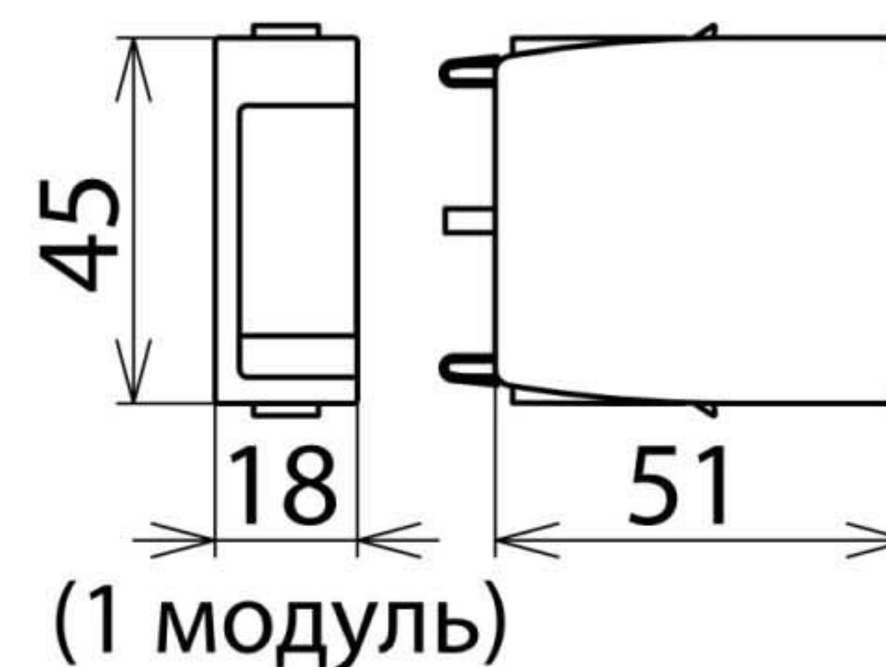
Размерный эскиз DG MOD 150
