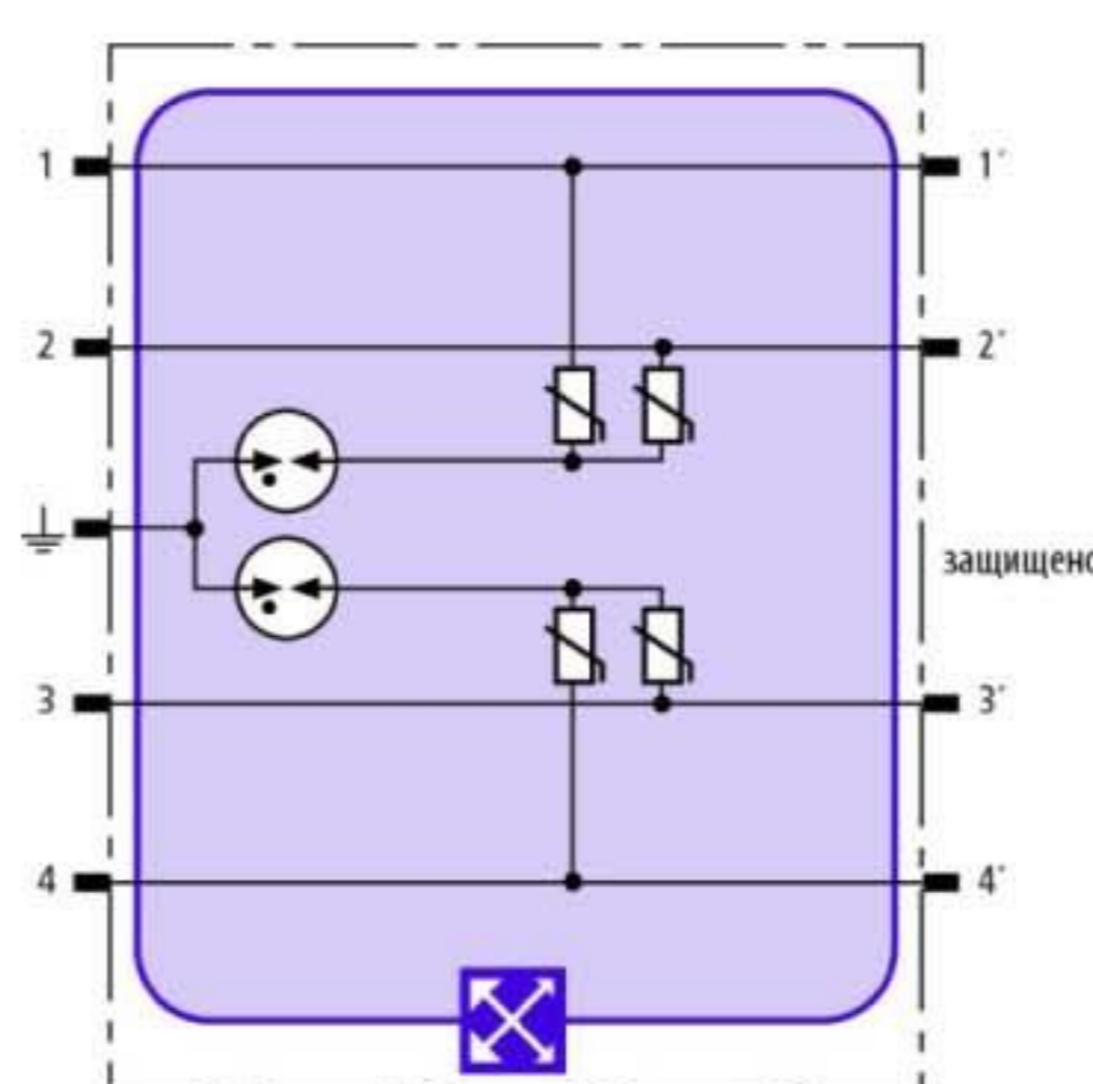
Принципиальная схема VXT ML4 MY 110
