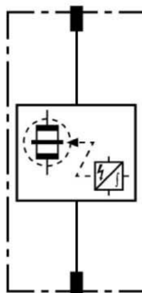
Принципиальная схема DSE MOD PE 60
