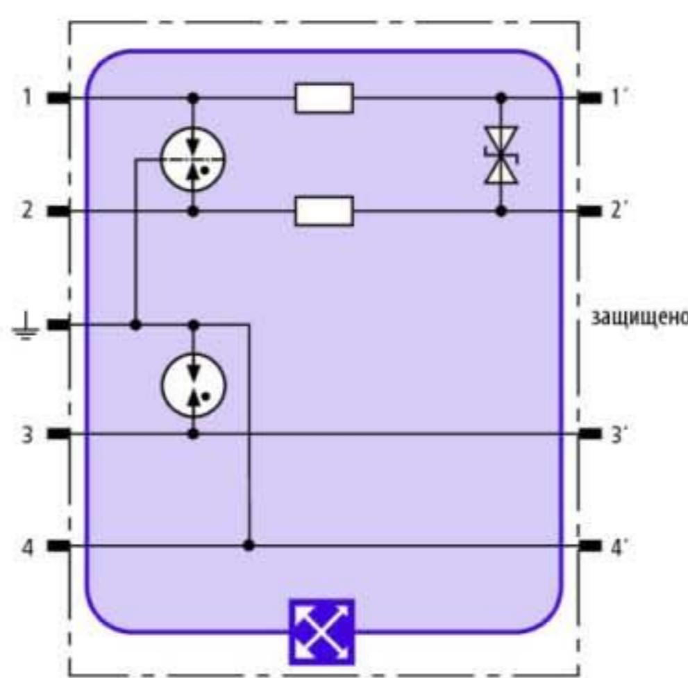
Принципиальная схема BXT ML2 BD S 12
