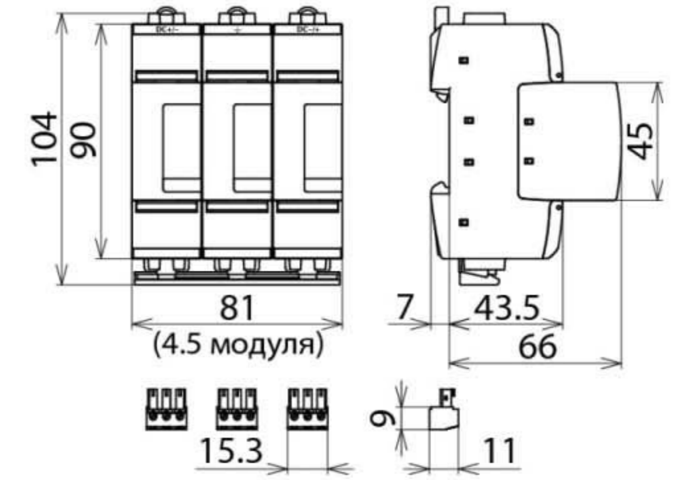
Размерный эскиз DG ME YPV SCI1500 FM
