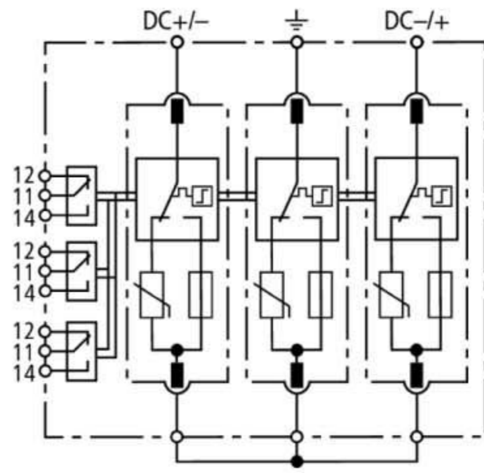
Принципиальная схема DG ME YPV SCI1500 FM
