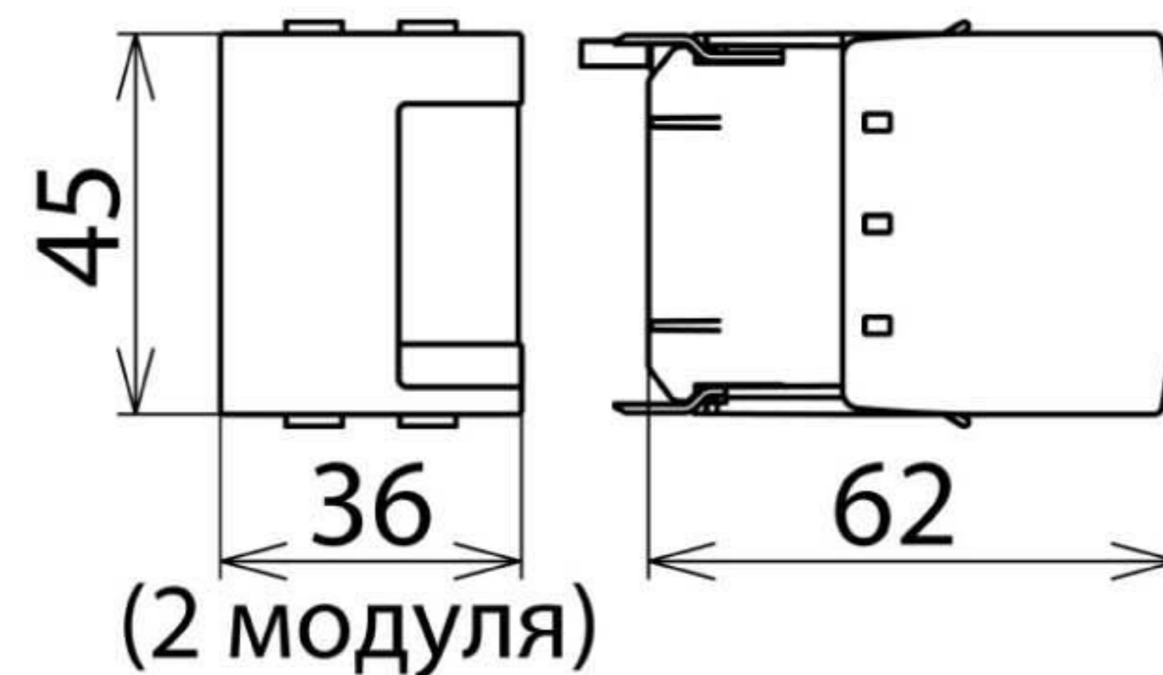
Размерный эскиз DSE MOD 60
