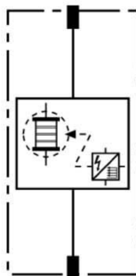
Принципиальная схема DSE MOD 60
