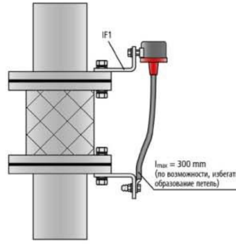
Пример монтажа EXFS L100
