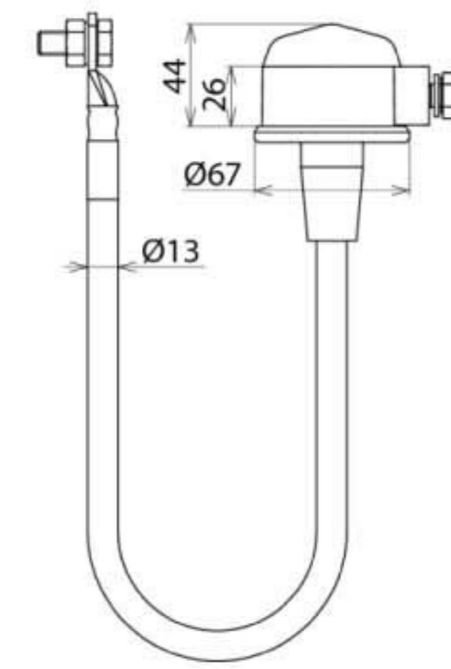
Размерный чертеж EXFS L100
