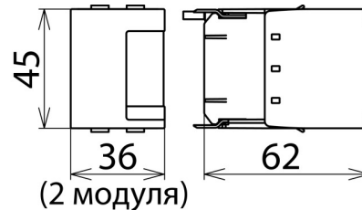
Размерный эскиз DSE MOD PE 60
