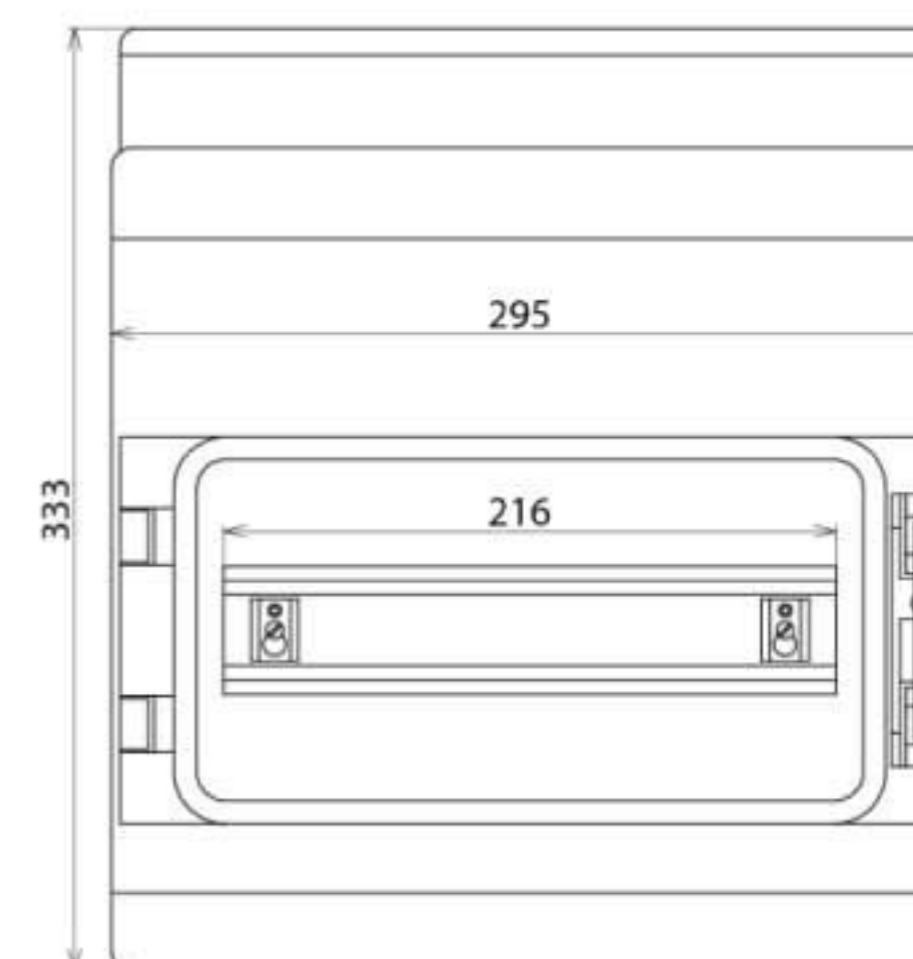
Размерный эскиз IGA 12 IP54
