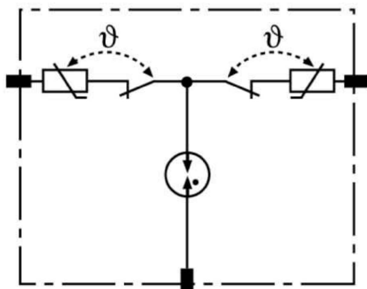
Принципиальная схема DR MOD 75
