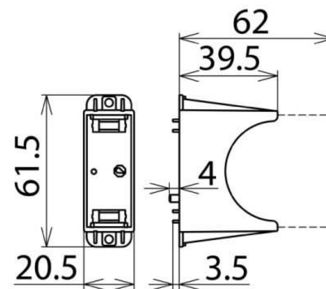
Размерный эскиз DG PCB PV SCI 500
