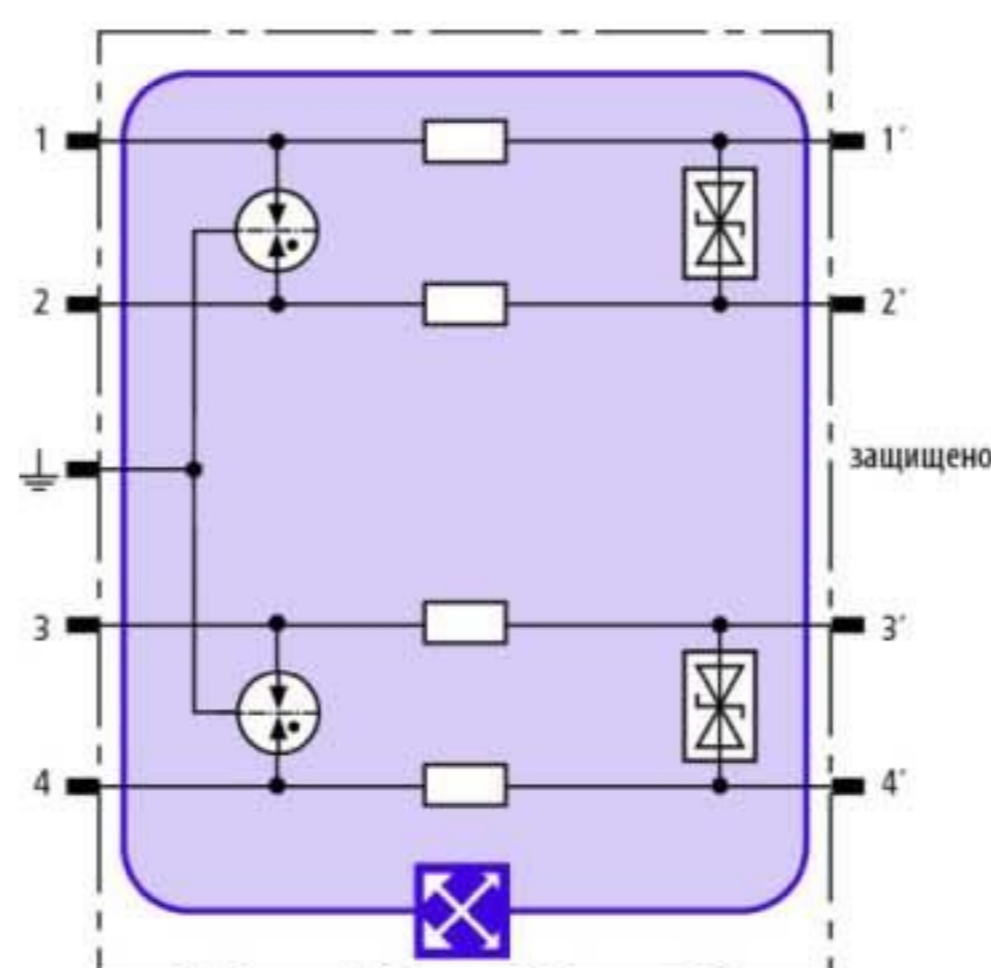
Принципиальная схема BXT ML4 BD HF 24
