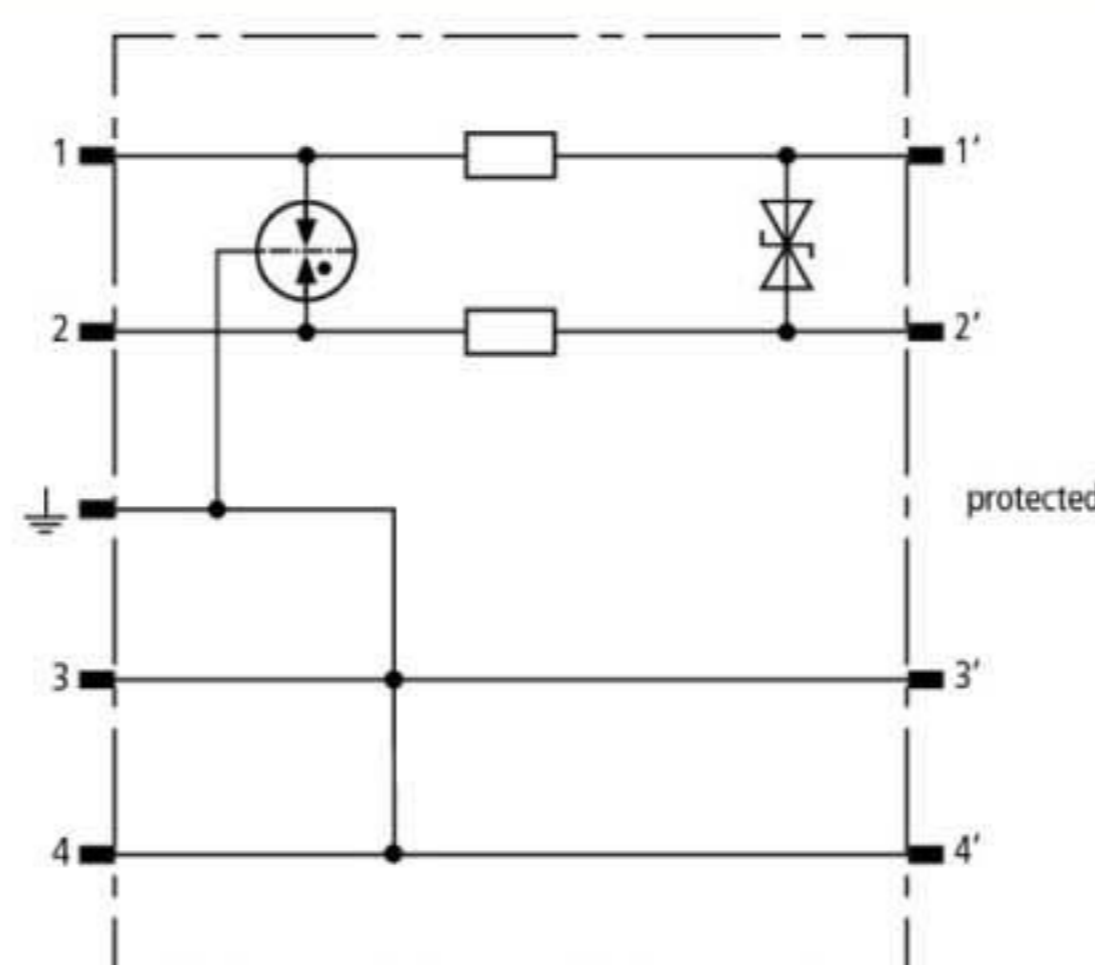
Принципиальная схема BSP M2 BD 12
