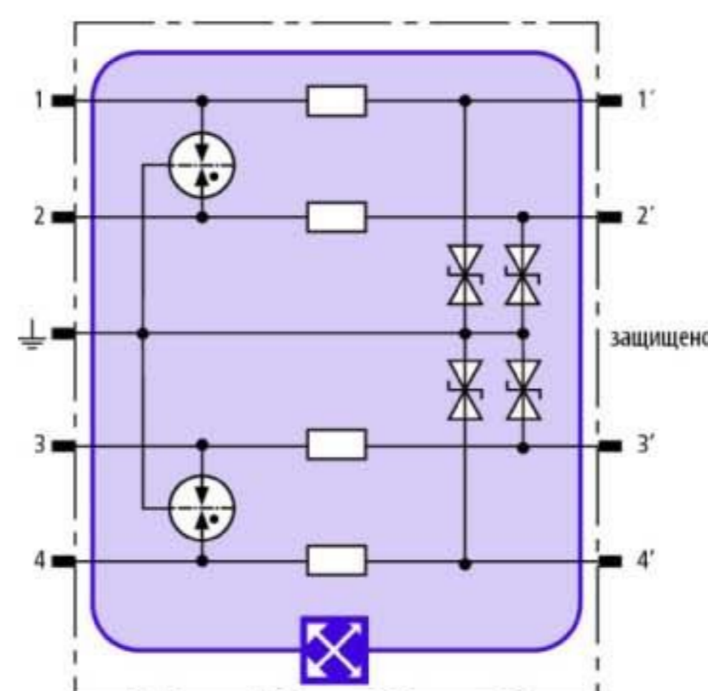
Принципиальная схема BXT ML4 BE 12
