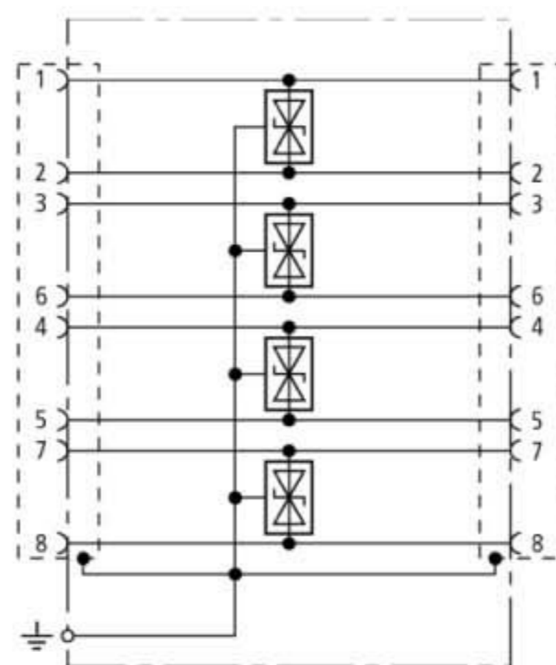
Принципиальная схема NET PRO 4TP 30
