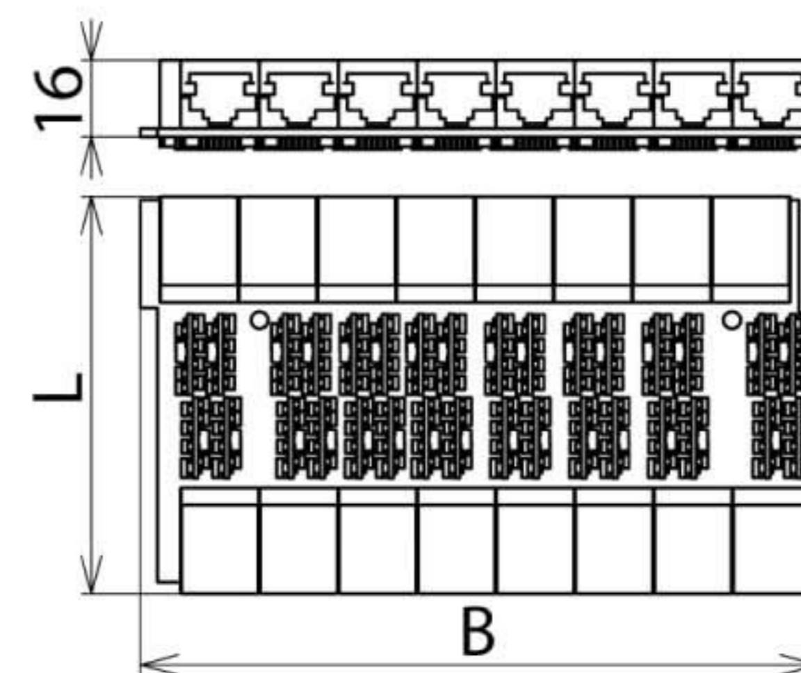
Размерный эскиз NET PRO 4TP 30
